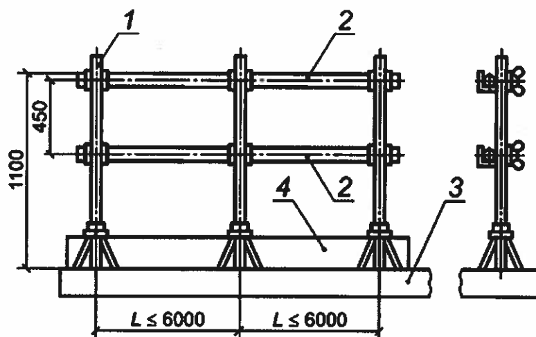
1 - стойка; 2 - заполнение; 3 - плита перекрытия; 4 - бортовая доска высотой 100 мм
