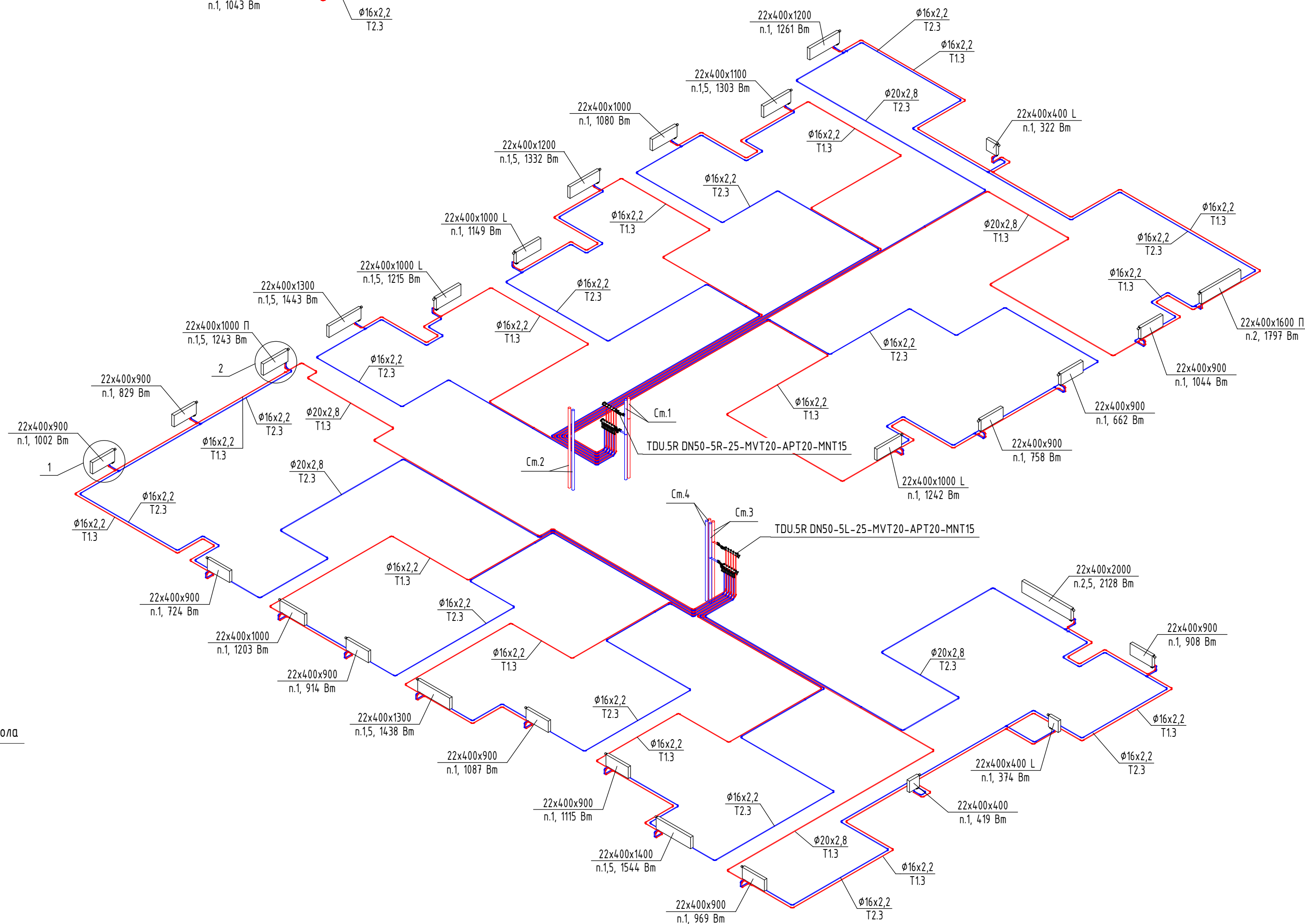
Схема системы отопления 4 этажа
