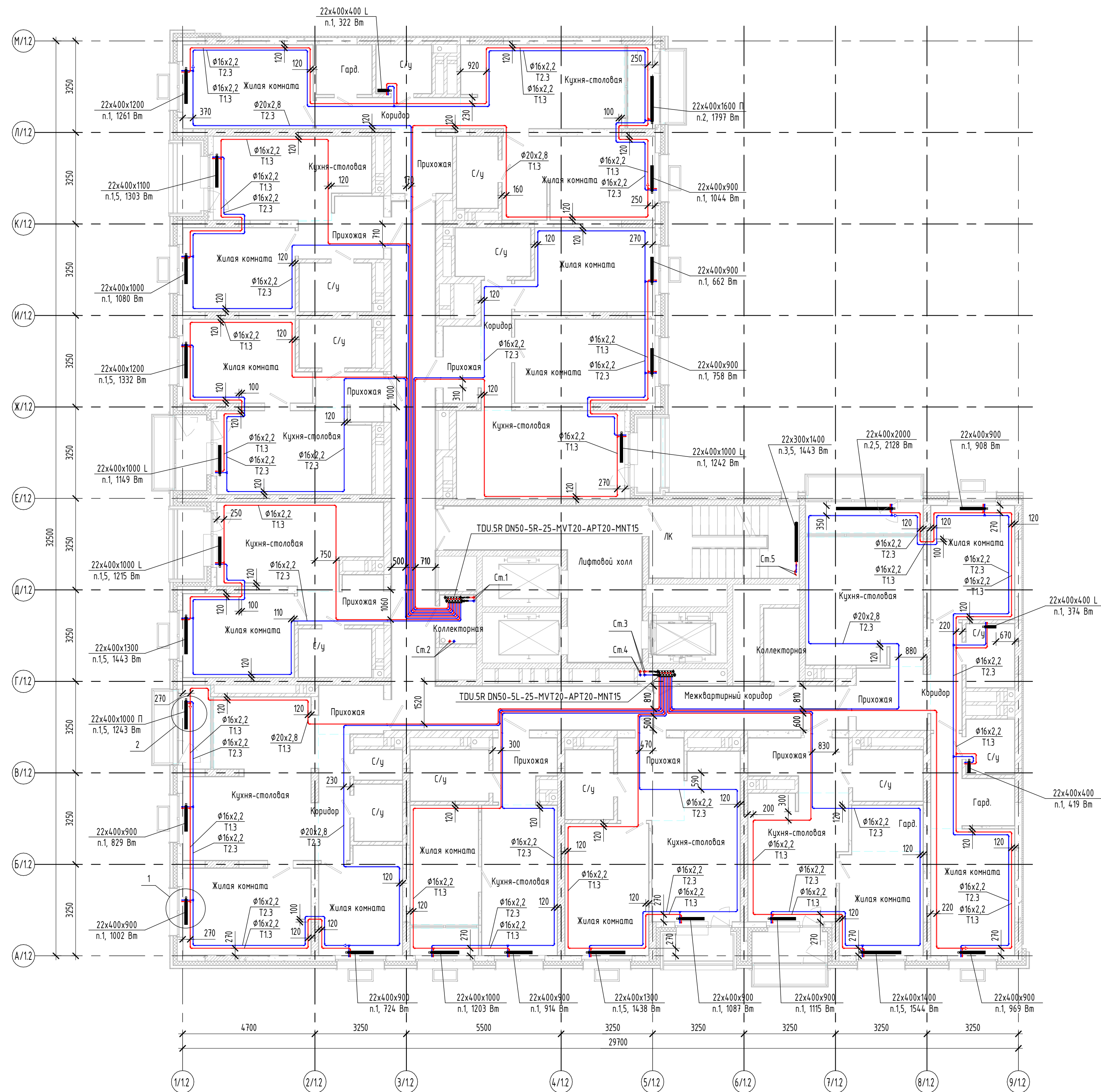
План 4 этажа
