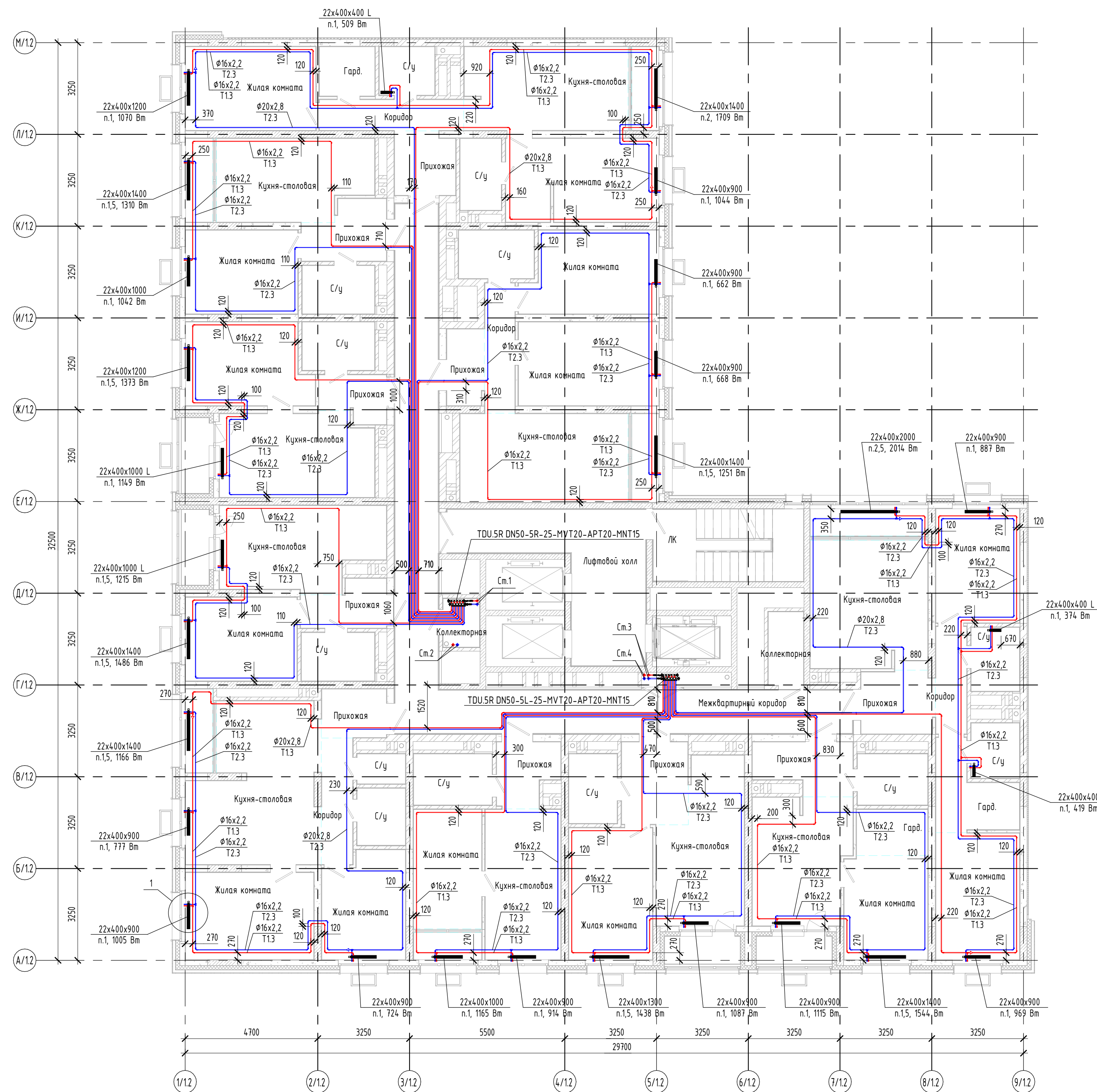
План 8 этажа
