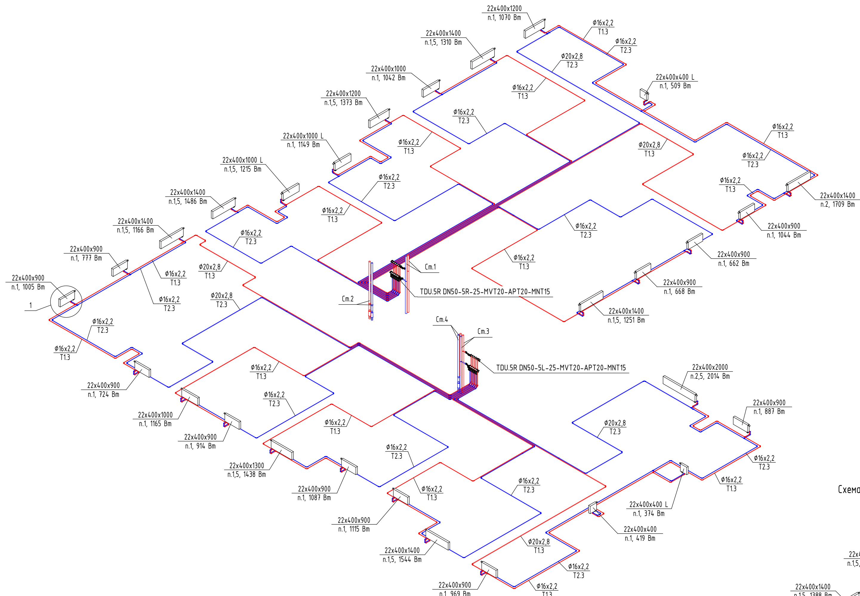
Схема системы отопления 8 этажа
