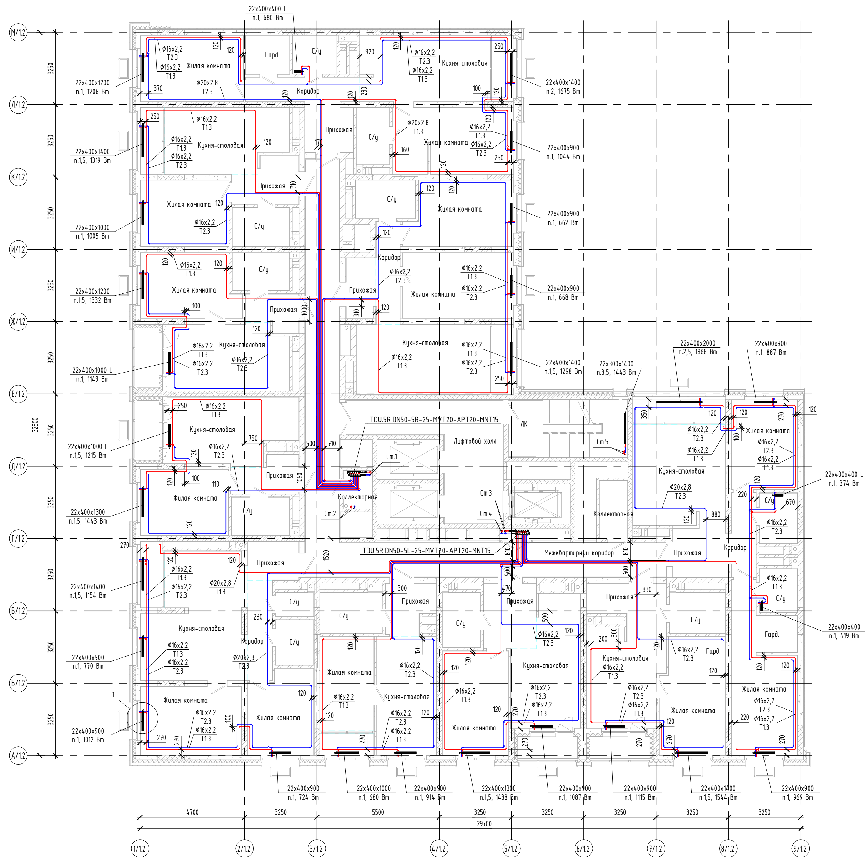
План 3 этажа
