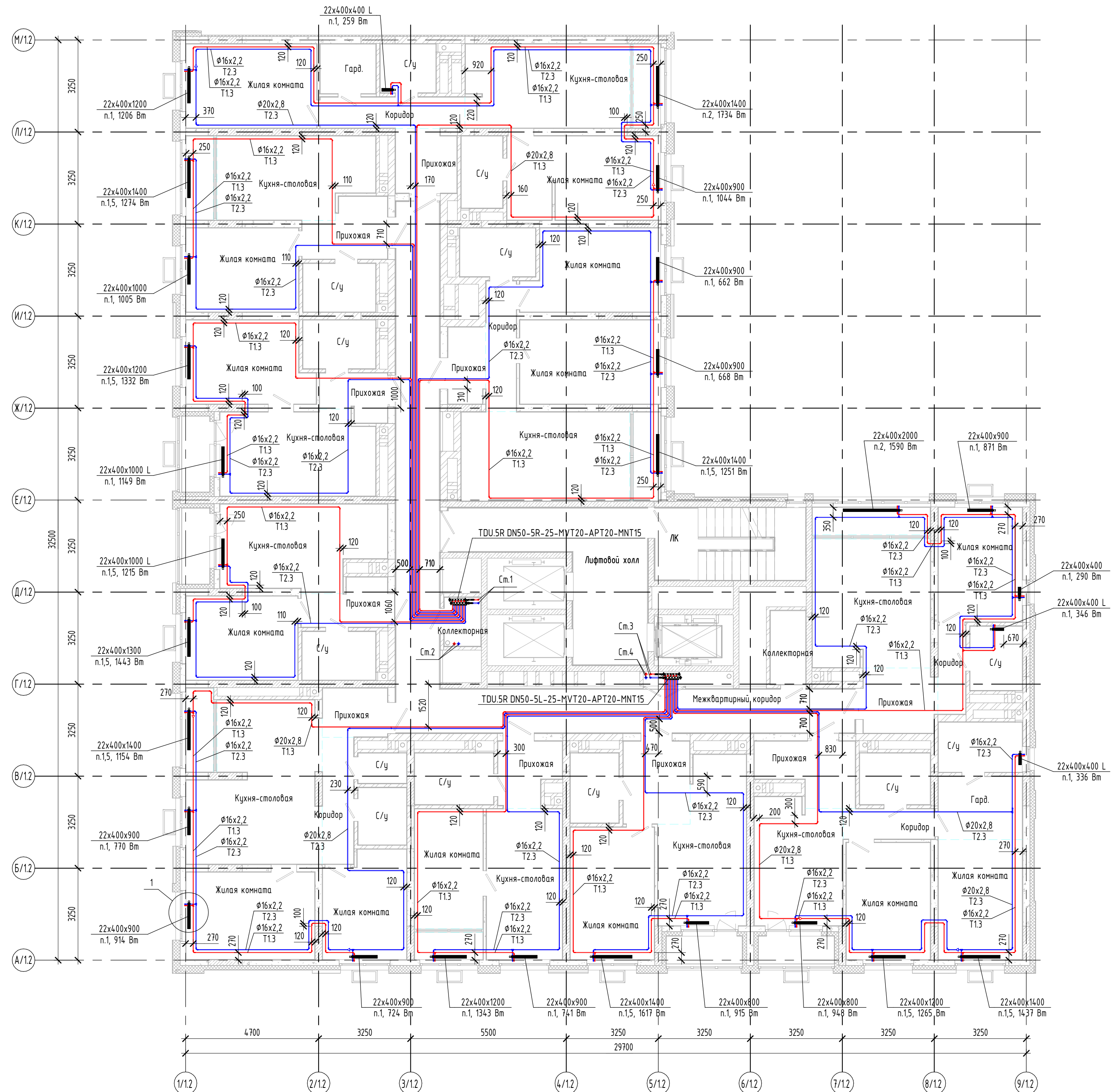
План 12-16 этажей
