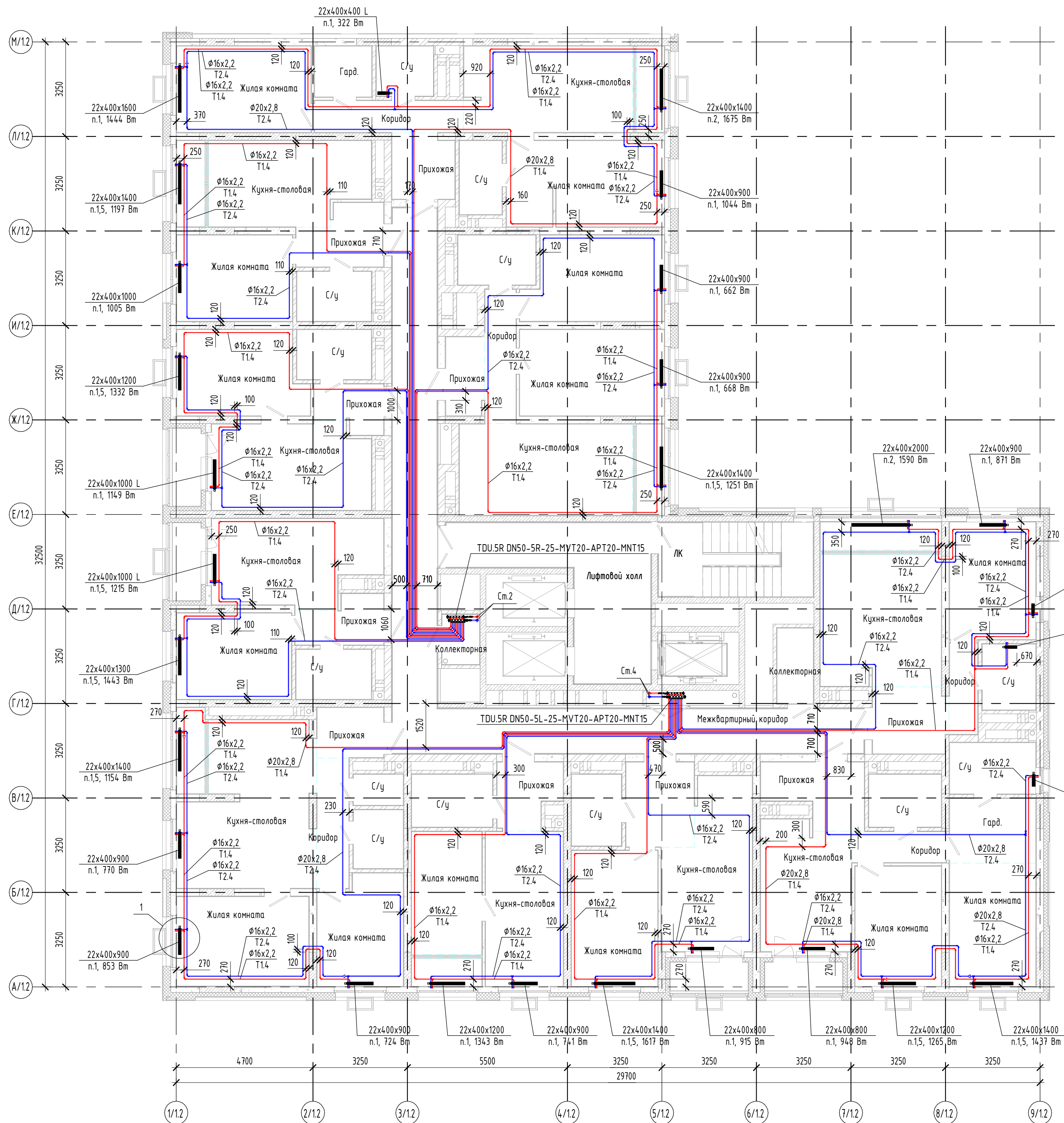
План 17-23 этажей
