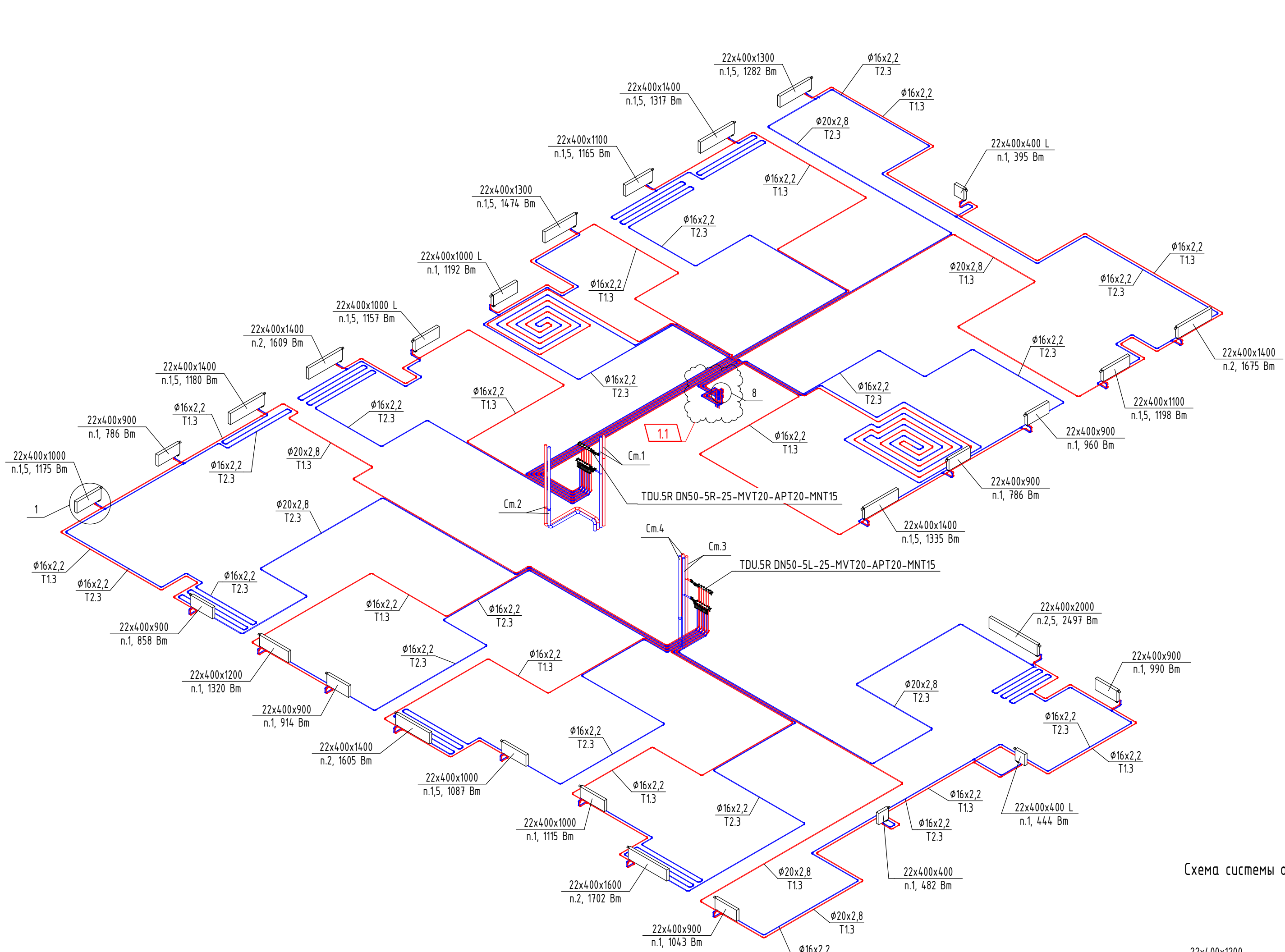
Схема системы отопления 2 этажа
