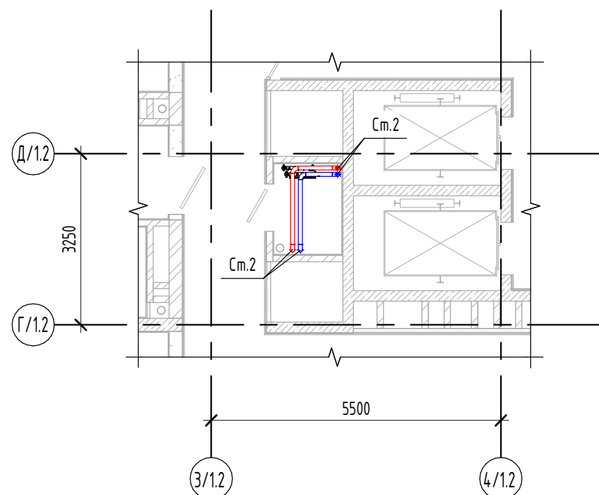
Фрагмент плана 14 этажа в осях Г/1,2 - Д/1,2, 3/1,2 - 4/1,2
