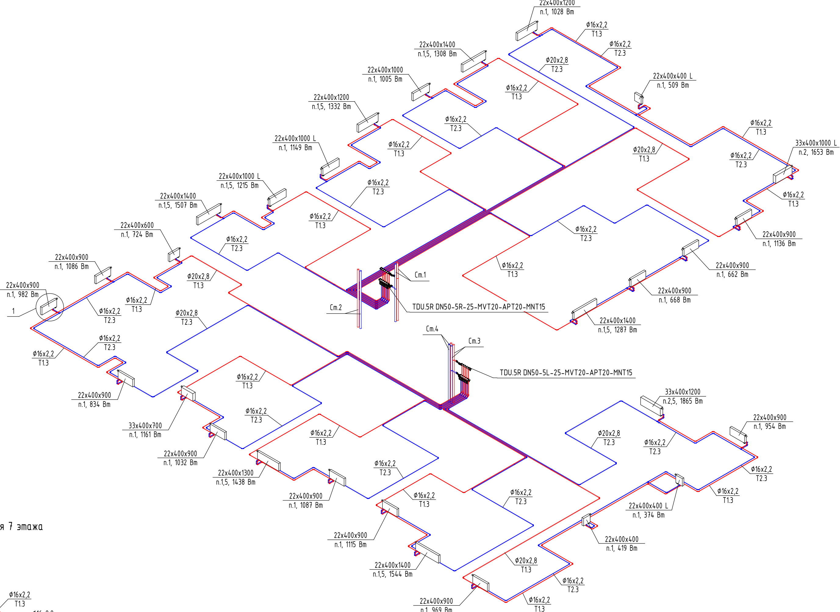
Схема системы отопления 6 этажа
