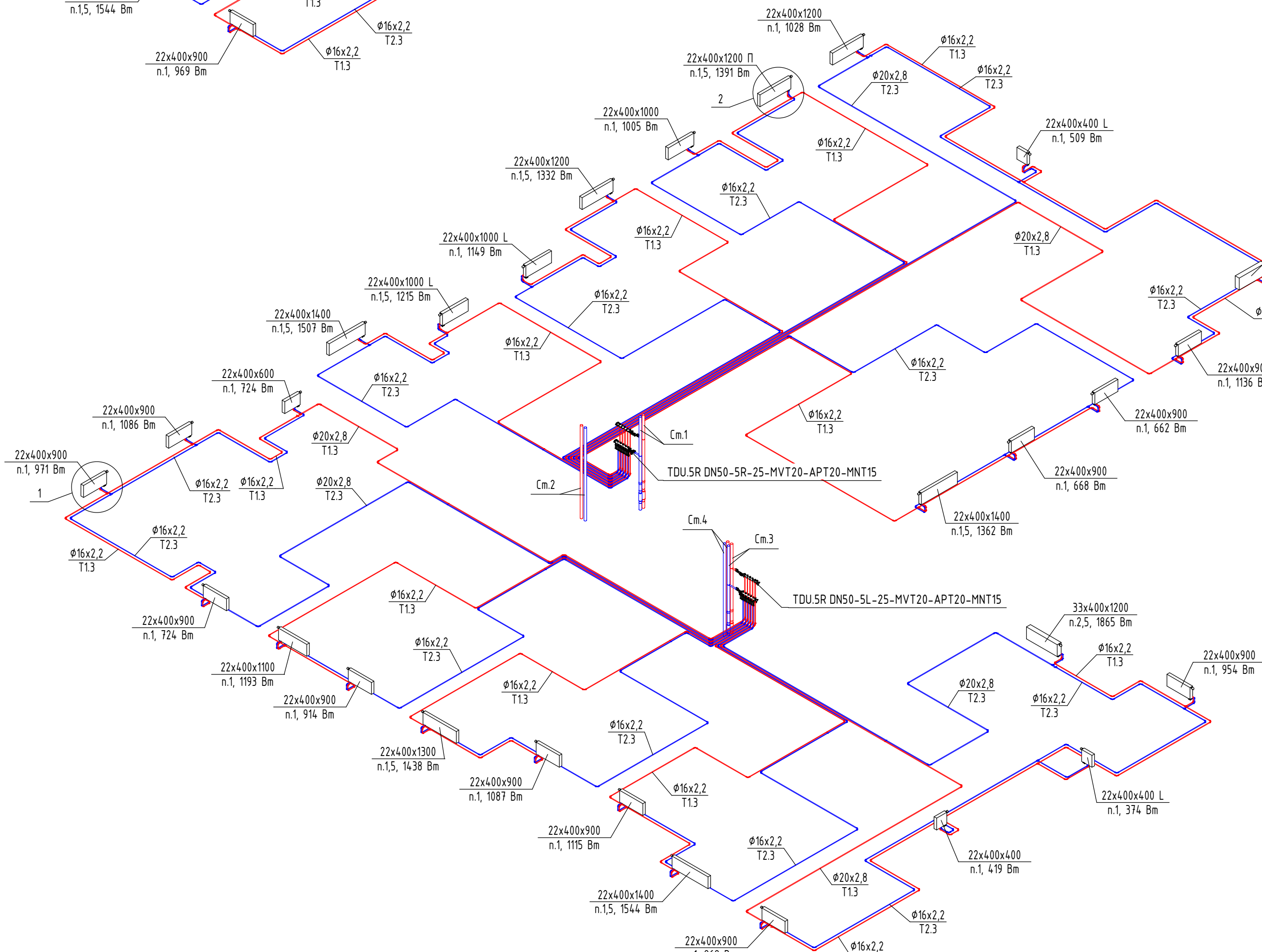
Схема системы отопления 7 этажа
