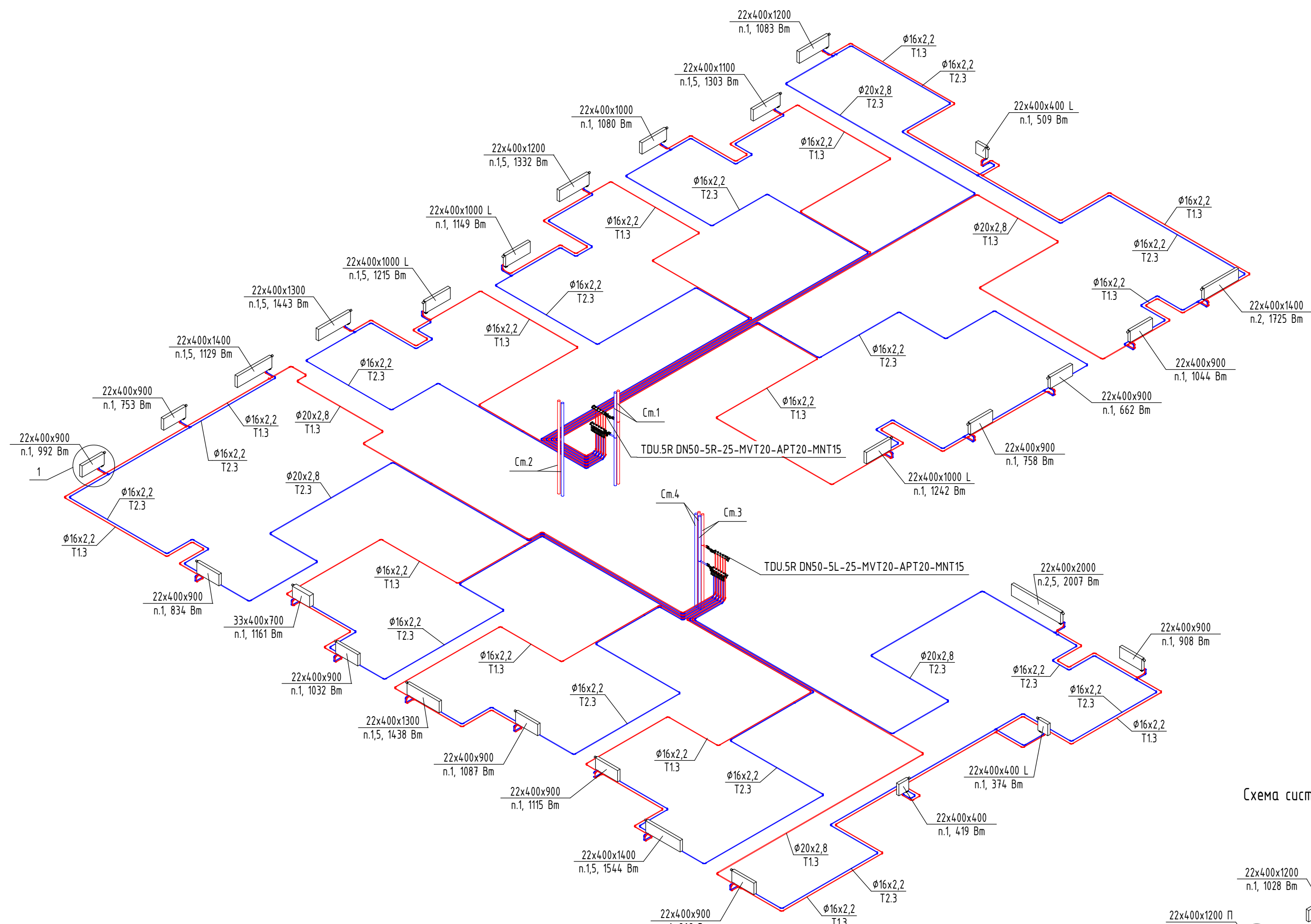
Схема системы отопления 5 этажа
