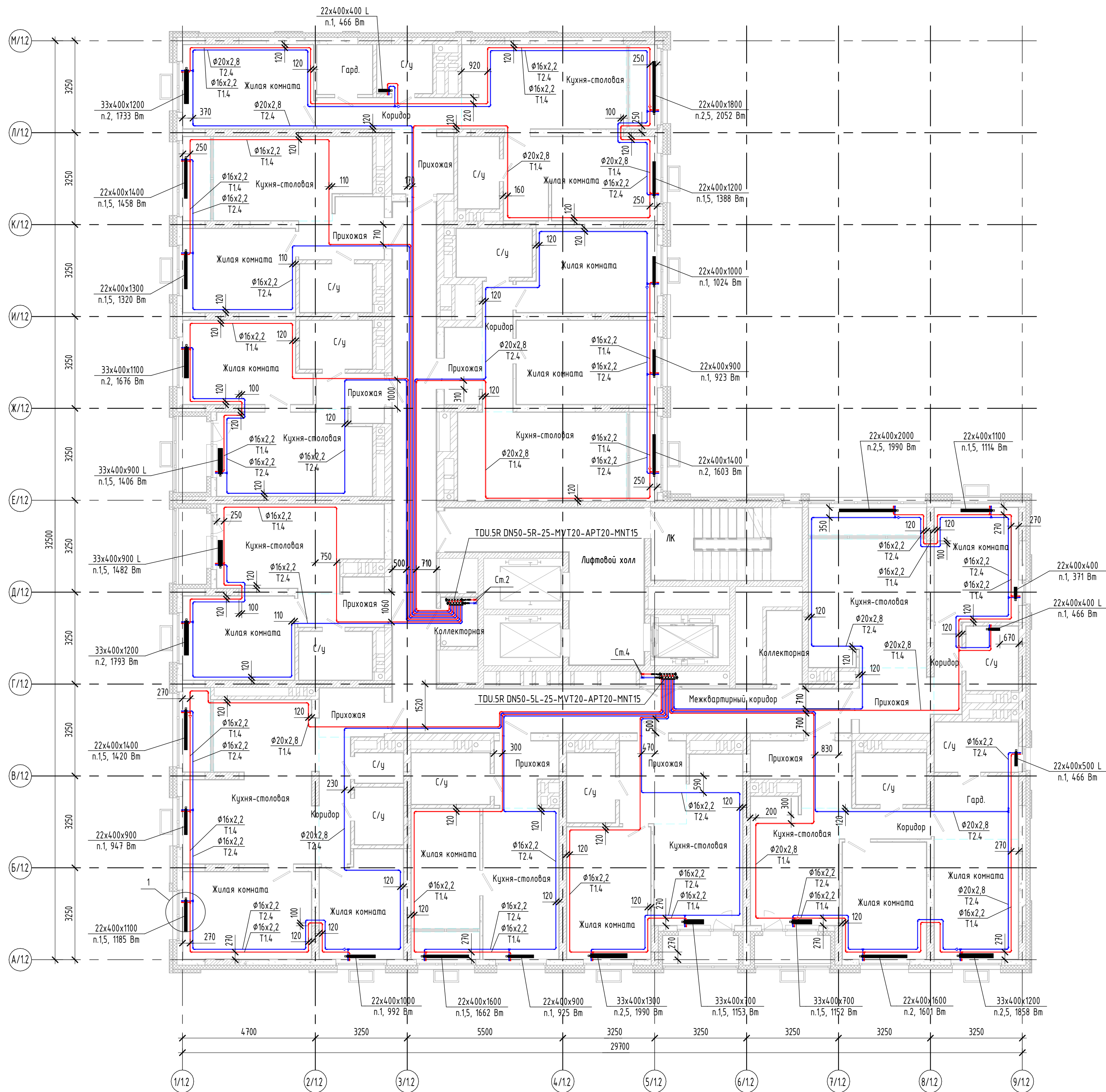
План 24 этажа
