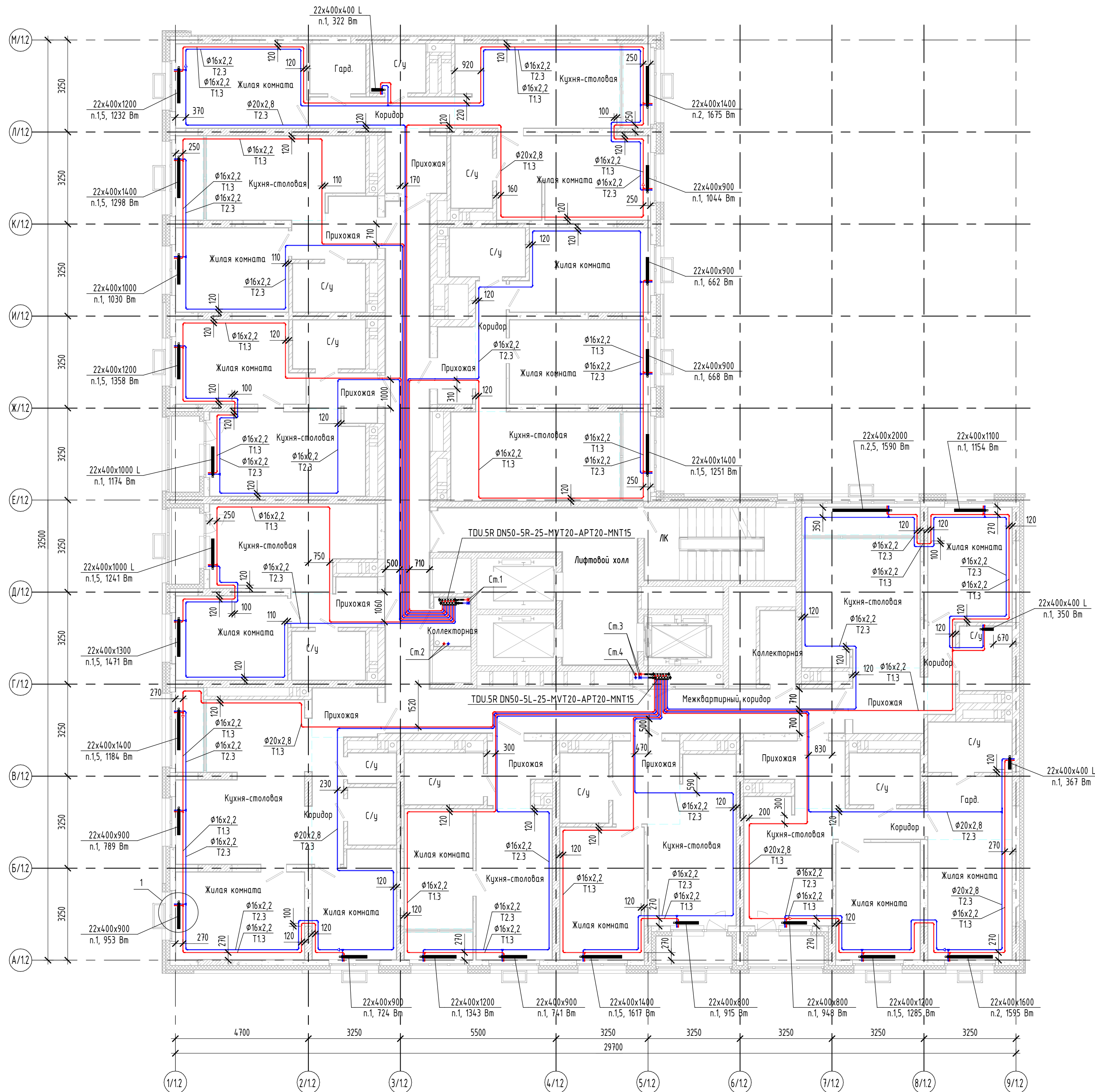
План 11 этажа
