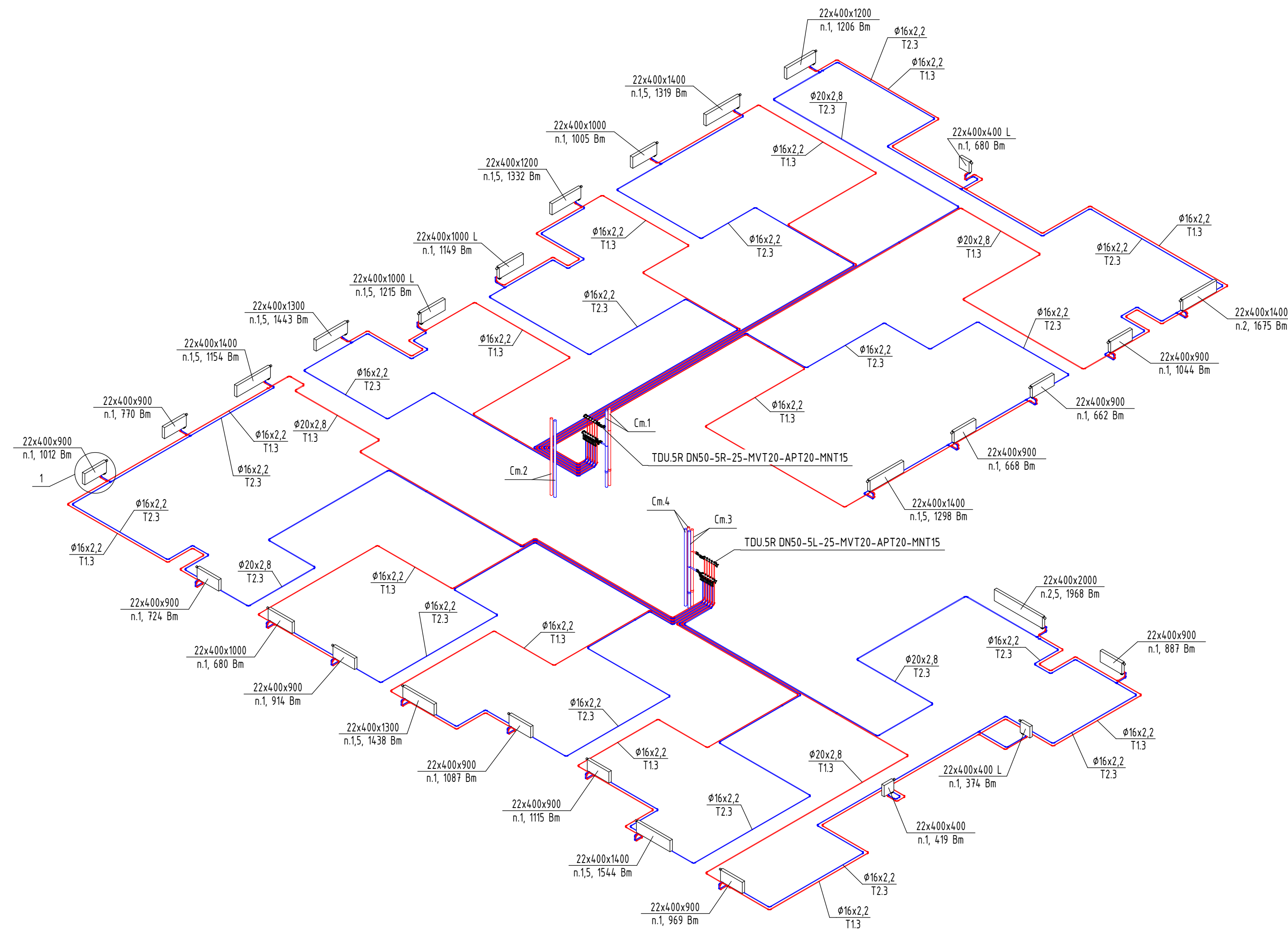
Схема системы отопления 4 этажа
