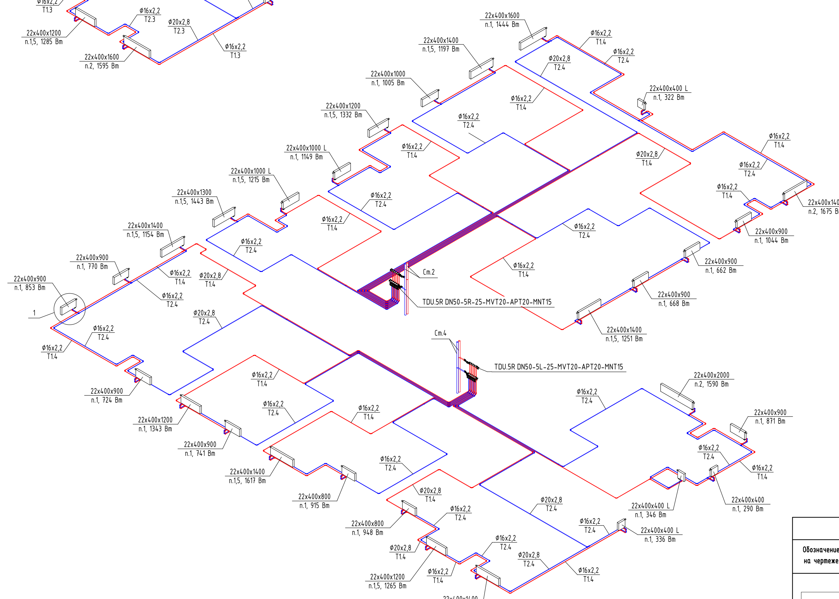
Схема системы отопления 17-23 этажей
