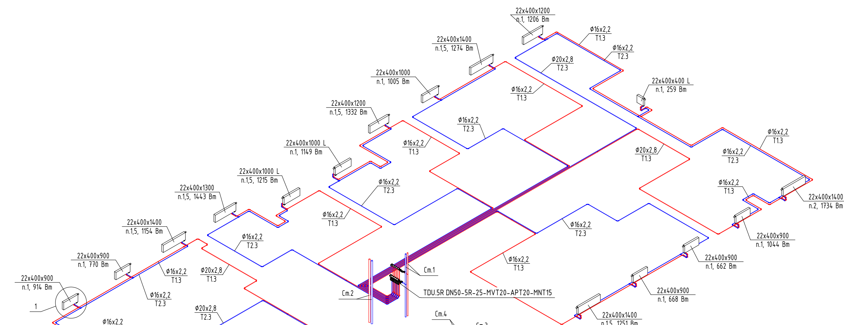
Схема системы отопления 12-16 этажей
