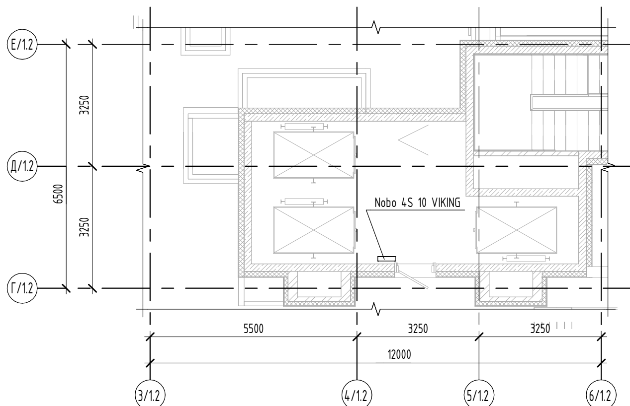
Фрагмент плана кровли в осях Г/1.2 - Е/1.2, 3/1.2 - 6/1.2
