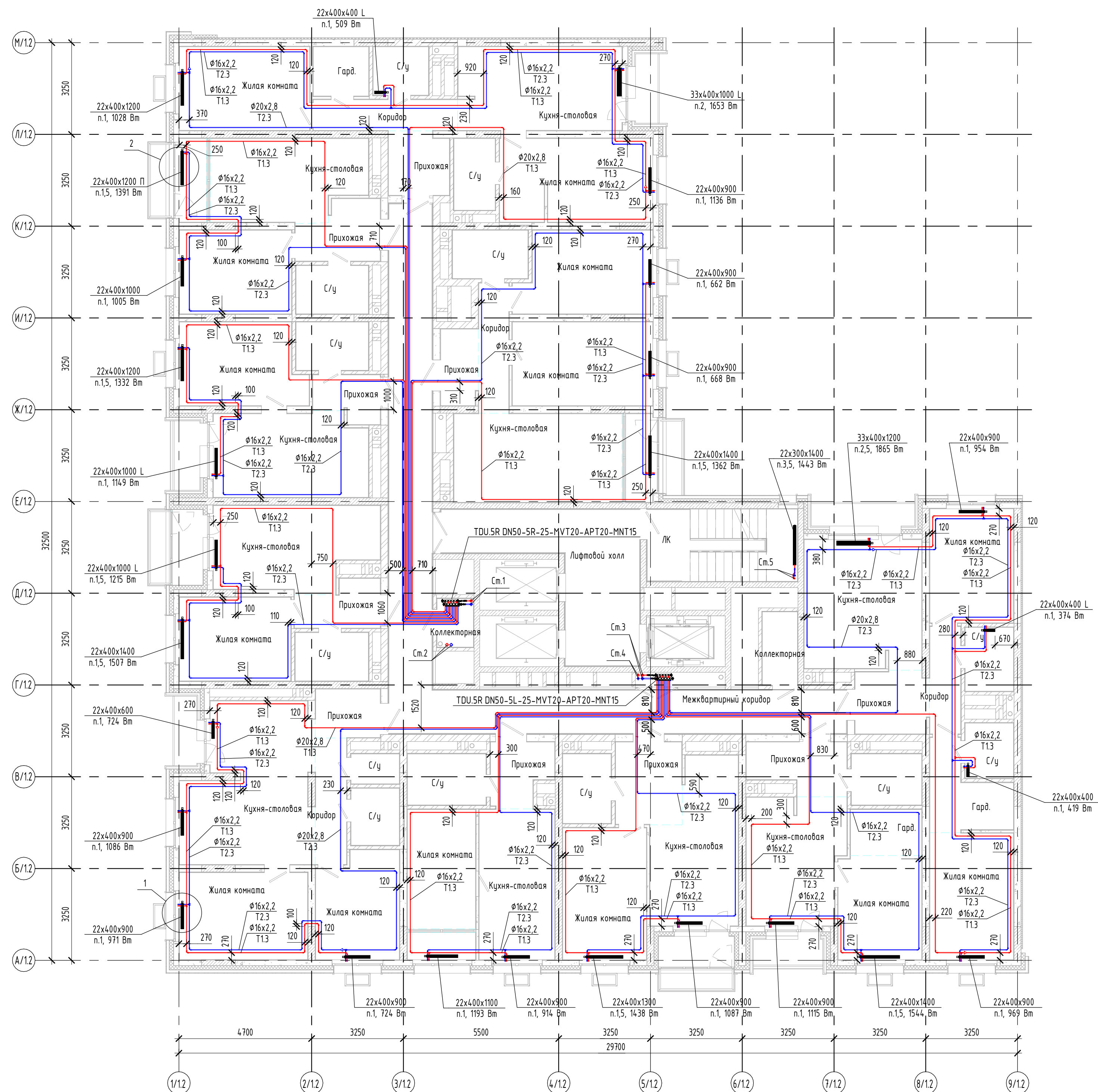
План 7 этажа
