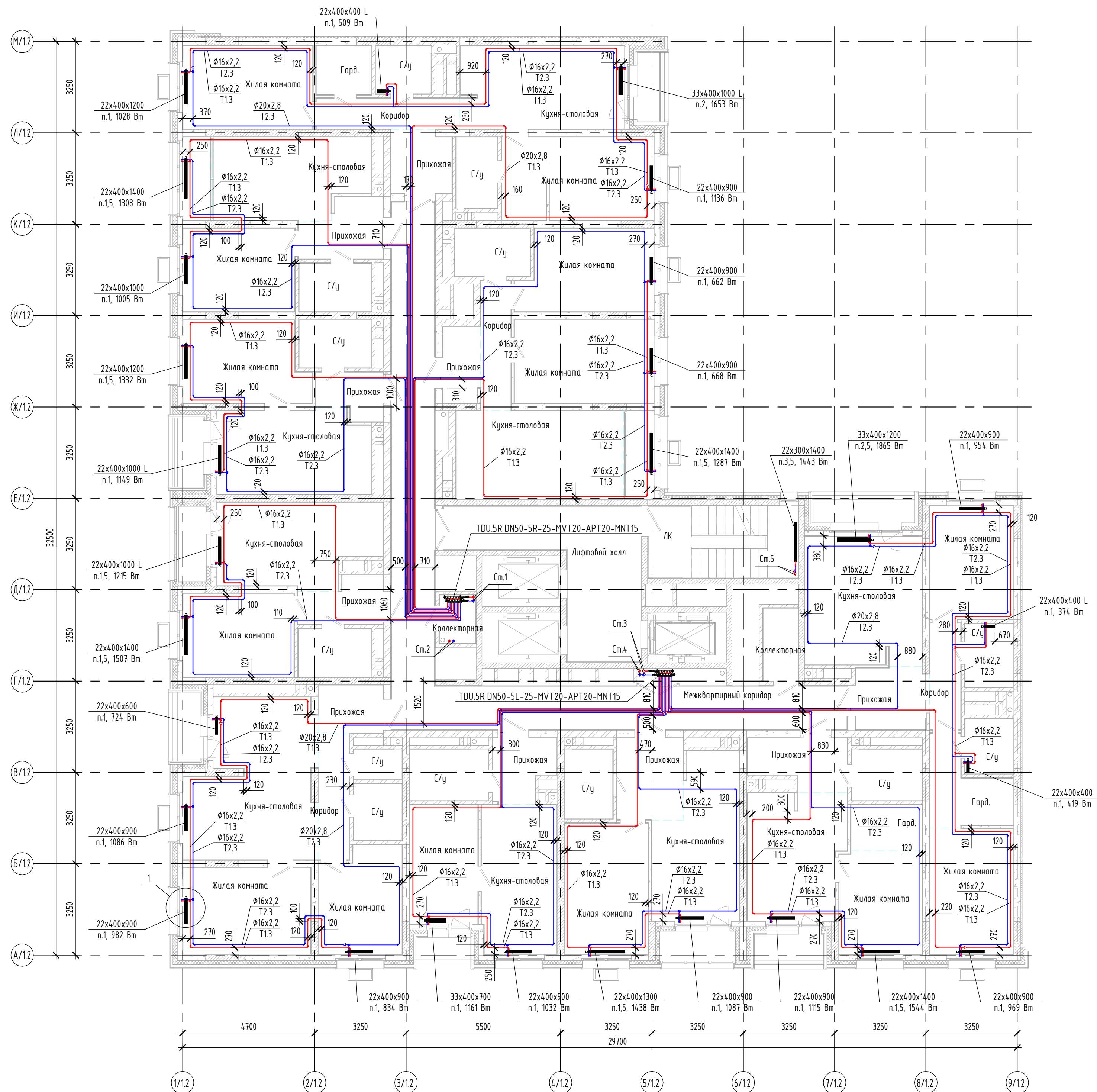
План 6 этажа
