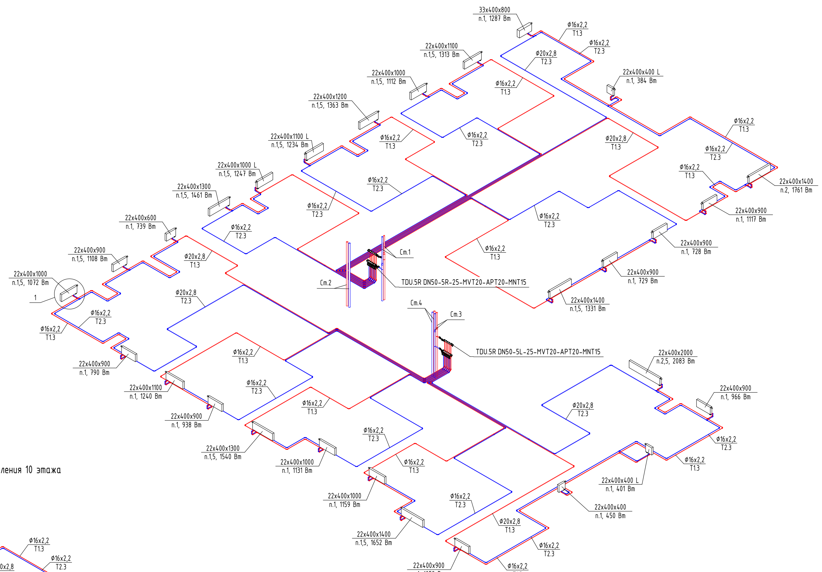
Схема системы отопления 9 этажа
