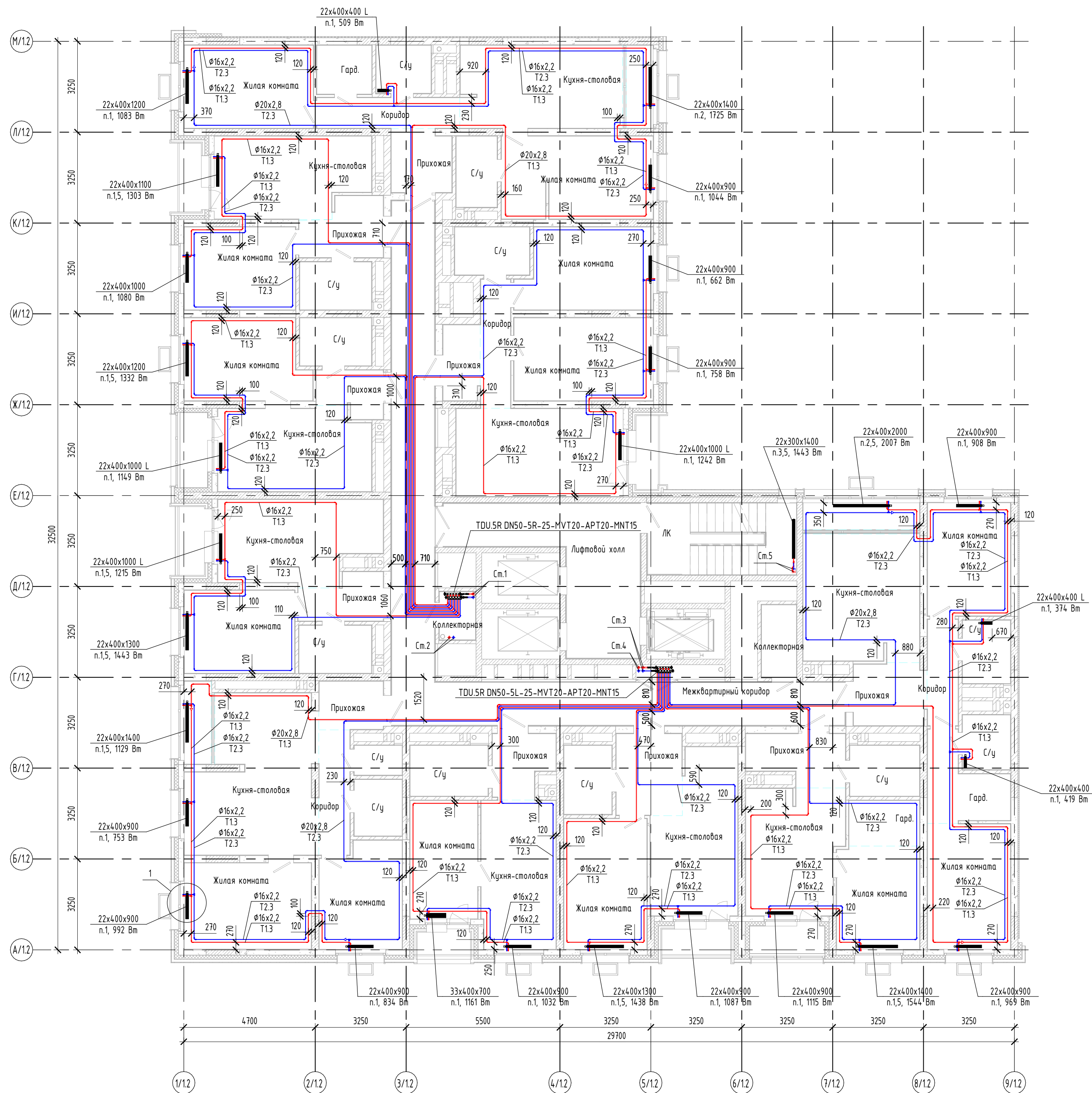
План 5 этажа
