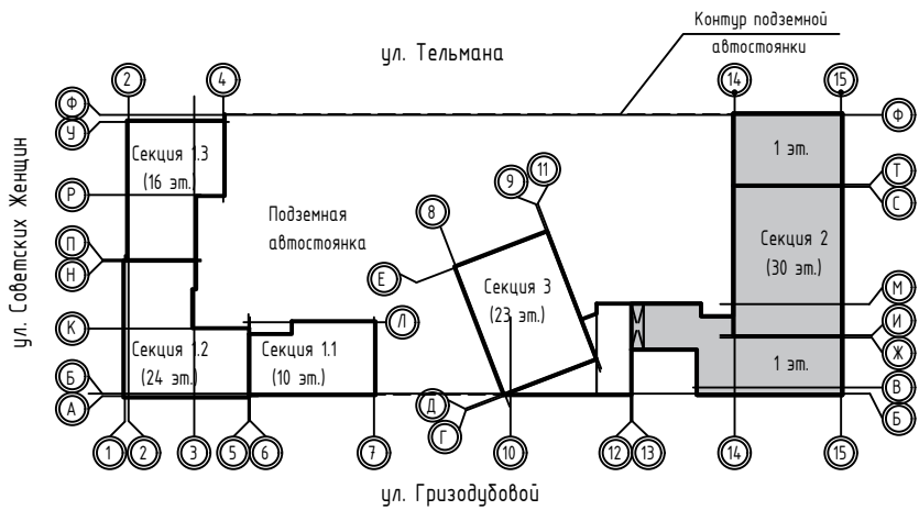
Блокировочная схема
