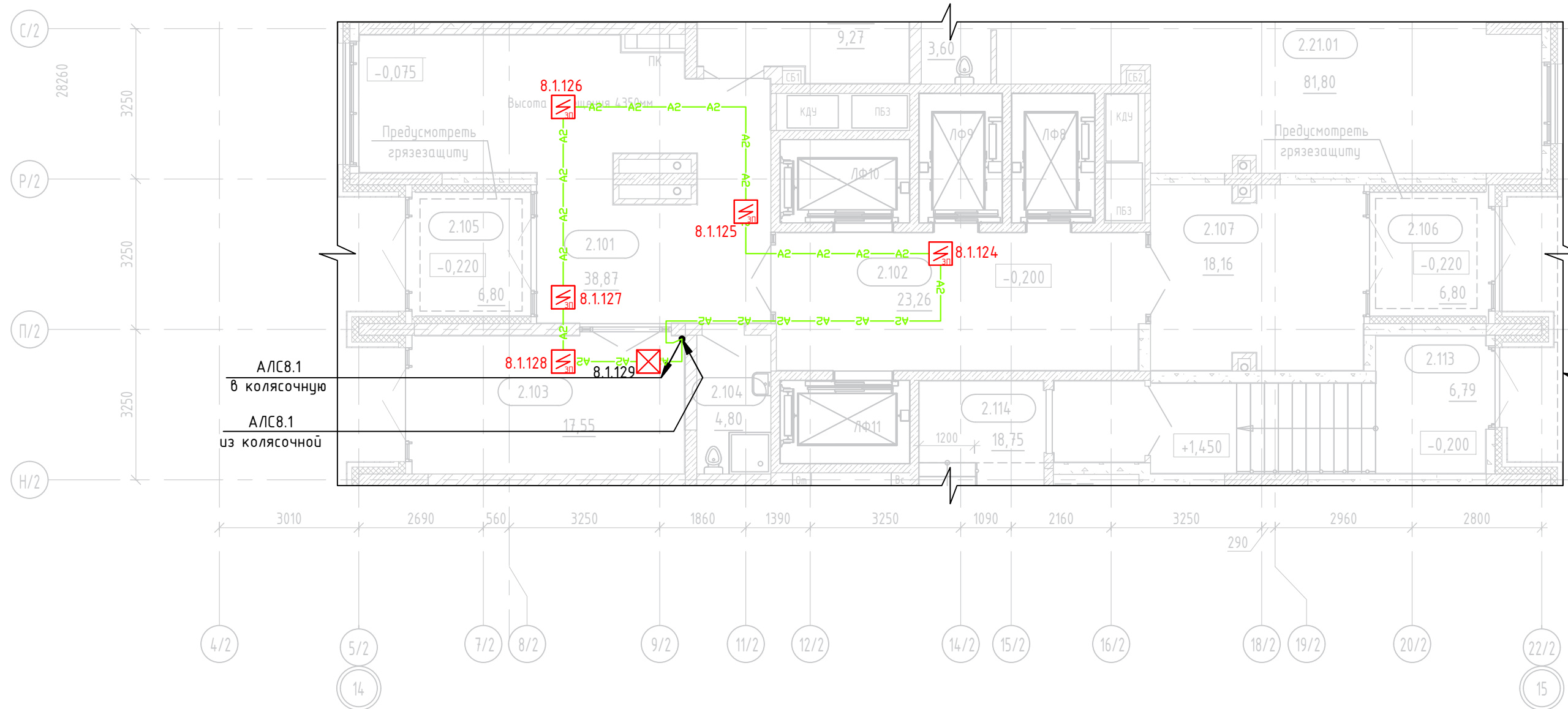
Фрагмент плана 1-го этажа (M1:100). Расстановка устройств в пространстве подвешенного потолка
