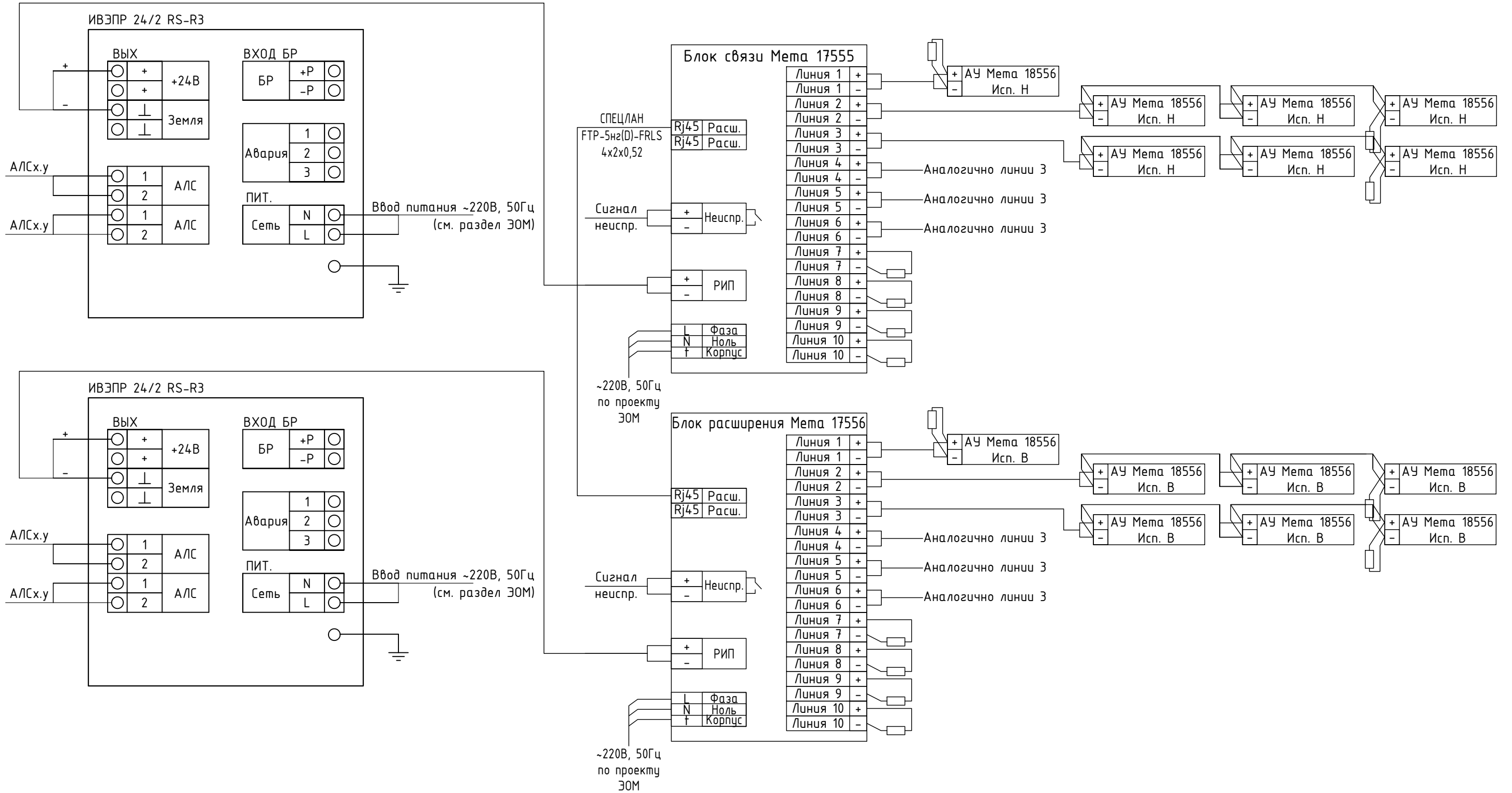
Типовая схема подключения оборудования системы двусторонней связи на базе оборудования Мета
