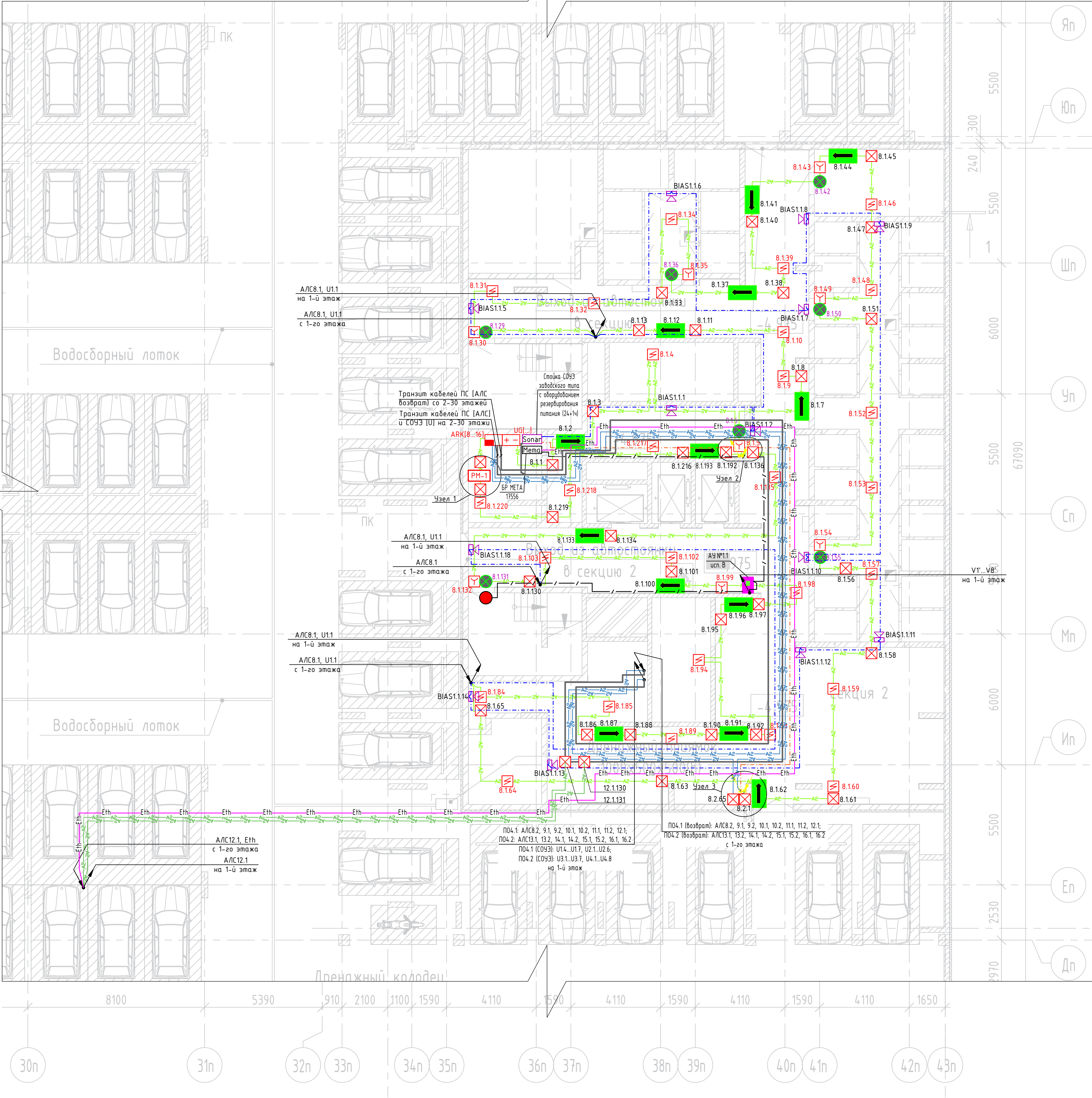
Фрагмент плана минус 1-го этаж под Секцией 2 (М1:100).
